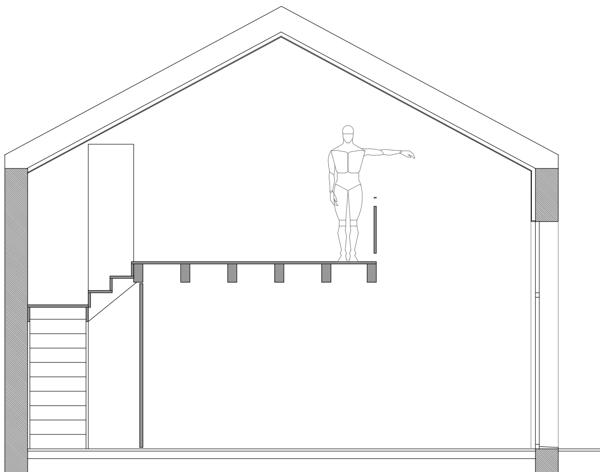
Corte 2-2
